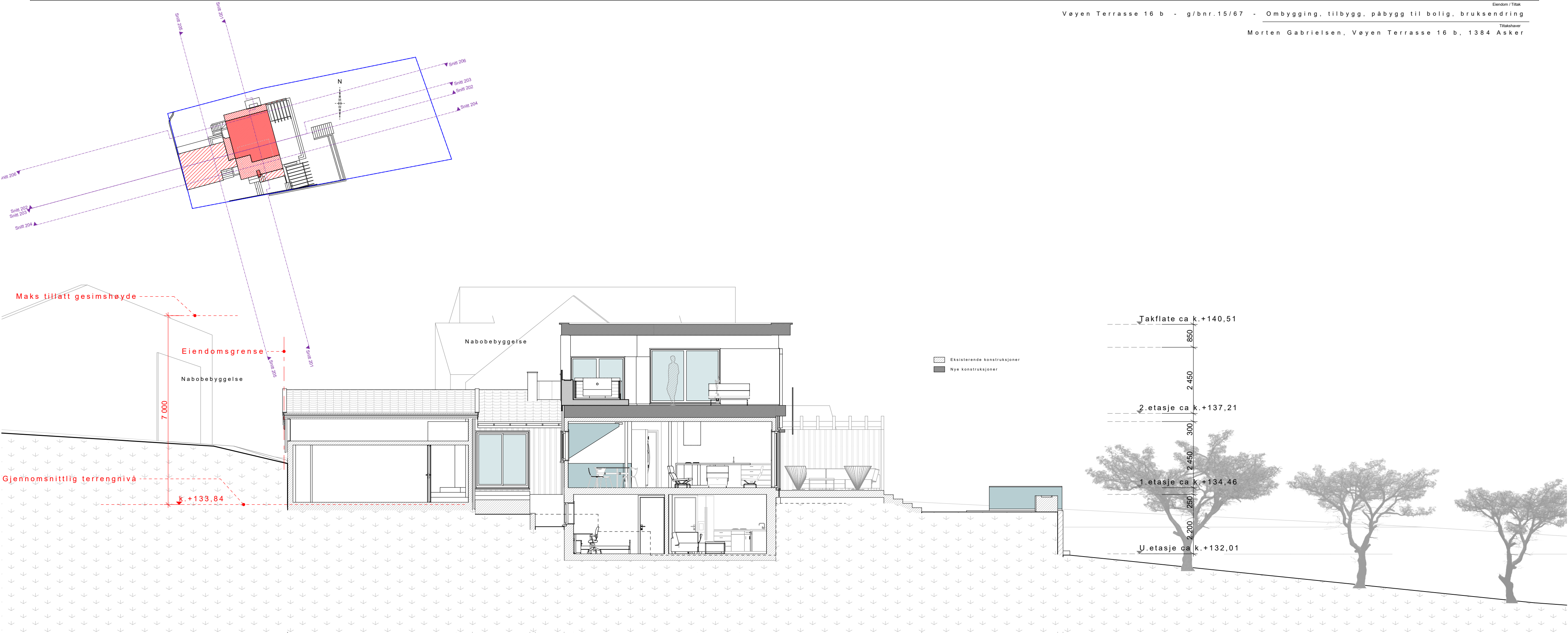
Snitt 204
