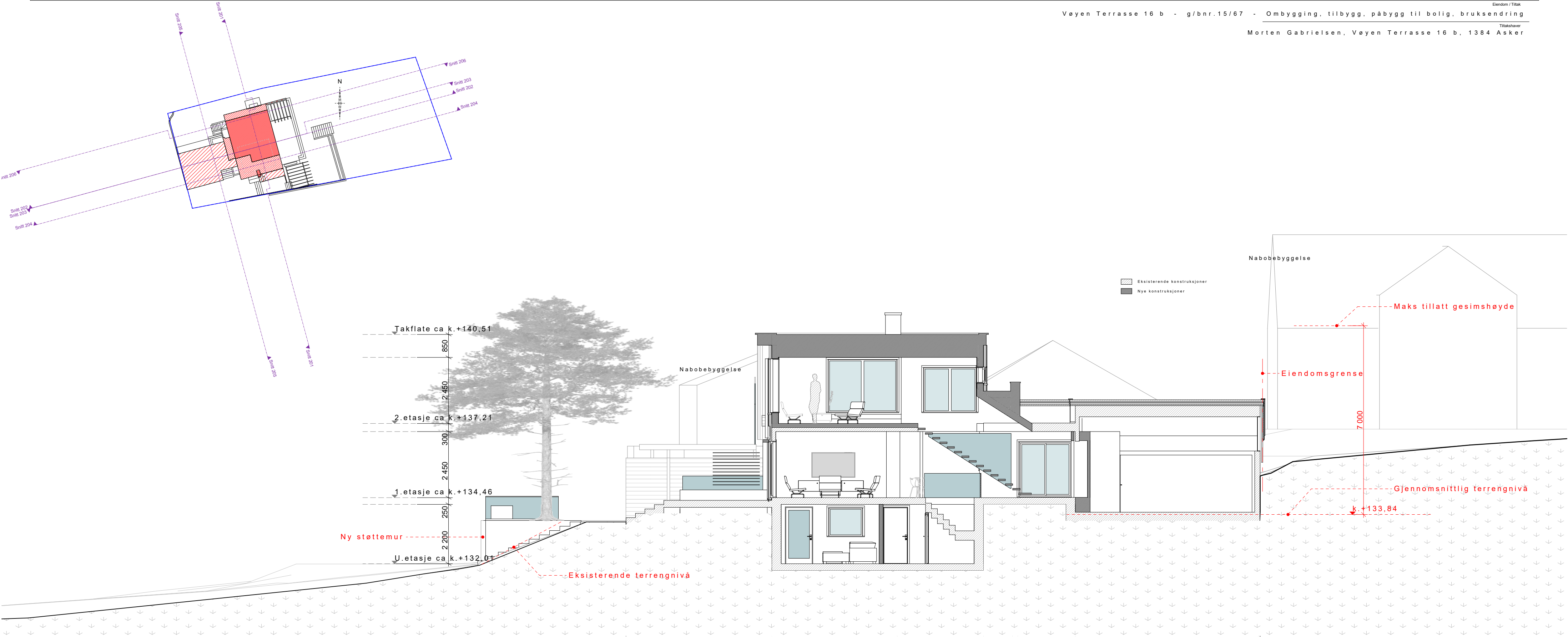
Snitt 203
