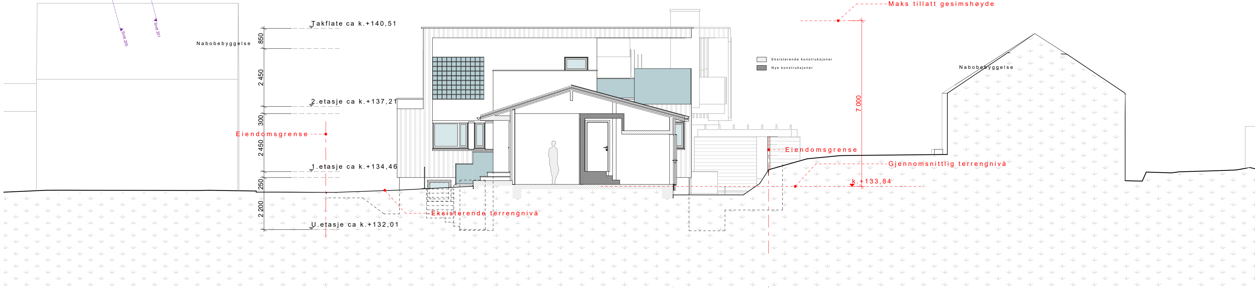
Snitt 205
